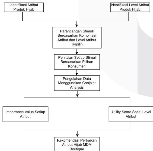
GAMBAR 2 Kerangka Konseptual
